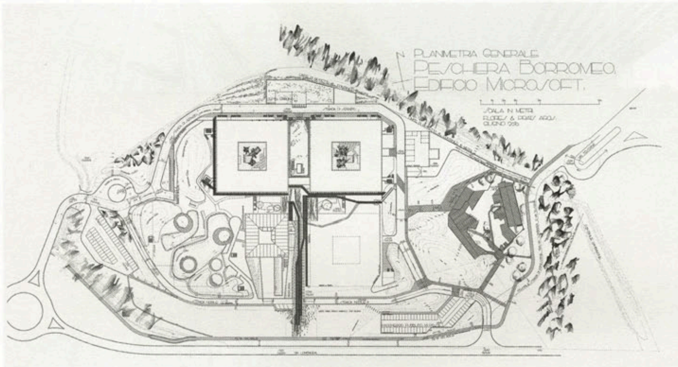
Planta de conjunt Planta de conjunto General plan
